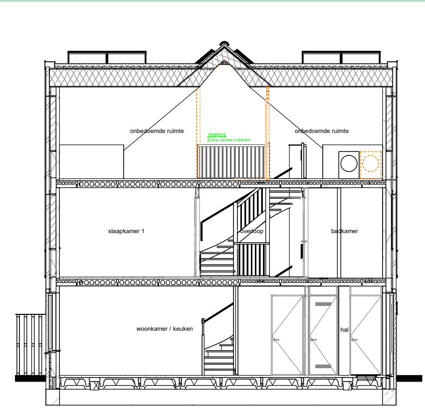
doorsnede zijkant
