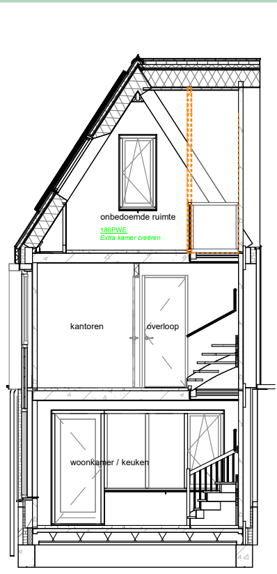
doorsnede voorkant
