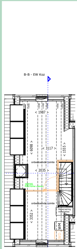
tweede verdieping
