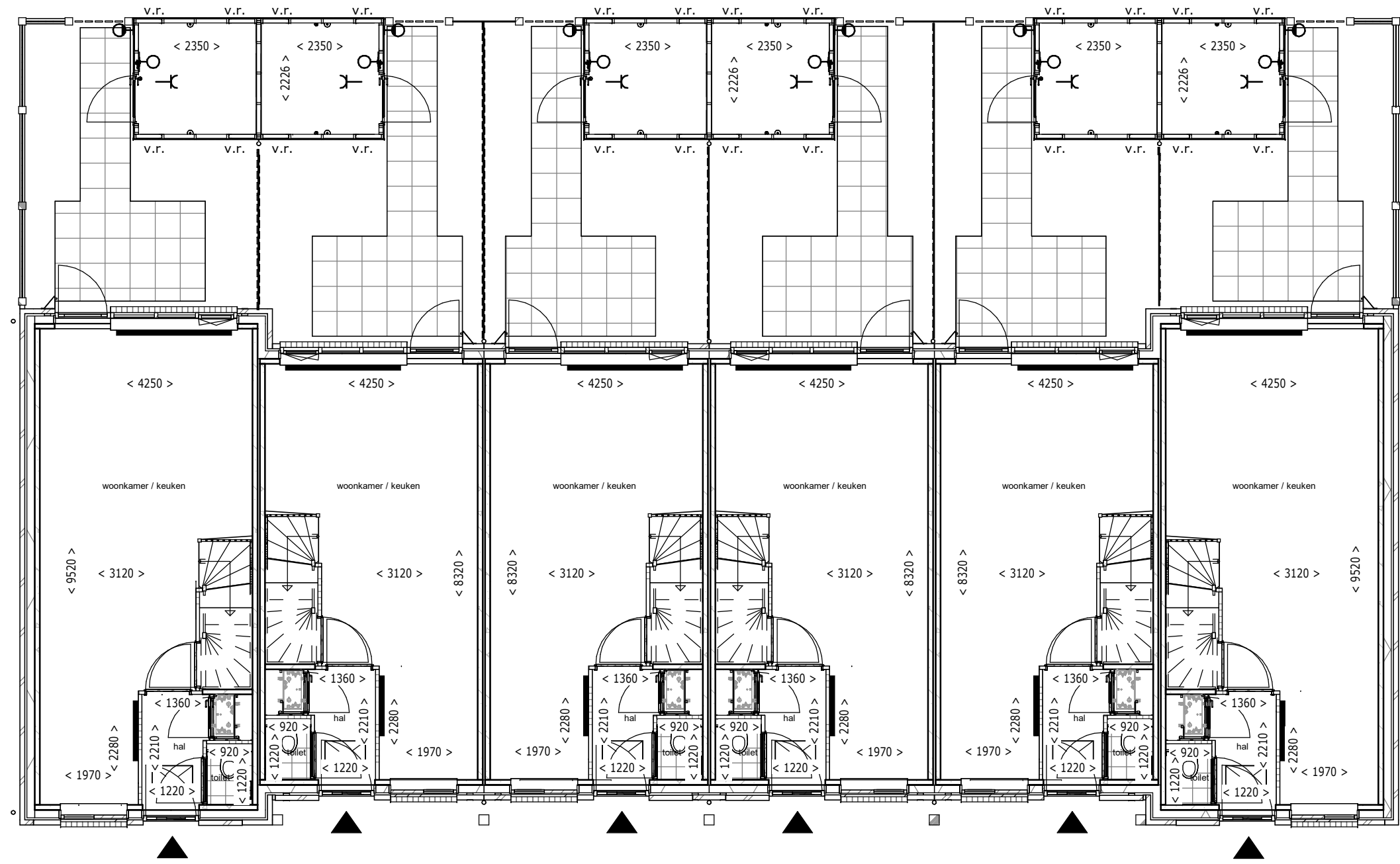
Begane grond - Blok 6
